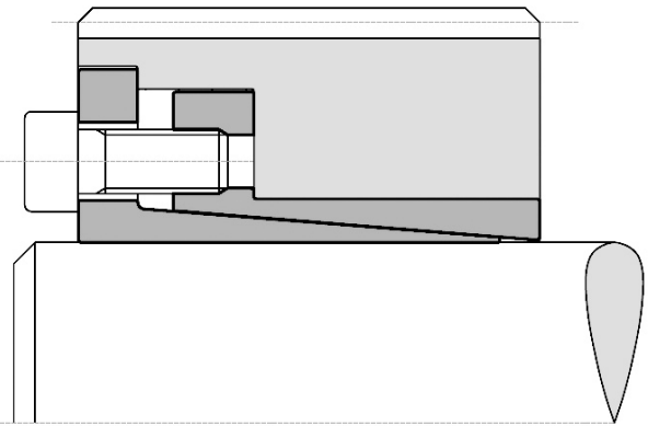
Sonderausführung TLK 132 mit Dichtringen
