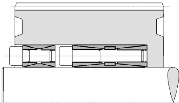
Sonderausführung TLK 132 mit Schutzring für die Schrauben
