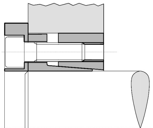
Sonderausführung TLK 132 mit Schutzring für die Schrauben
