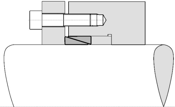
Anwendung TLK 110 bei hoher Drehzahl
