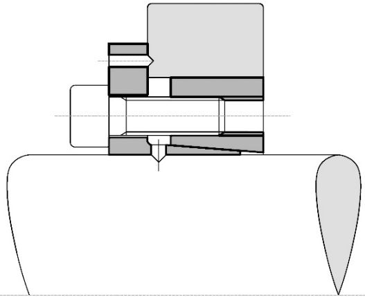
Sonderausführung TLK 133 für Nockenbefestigung
