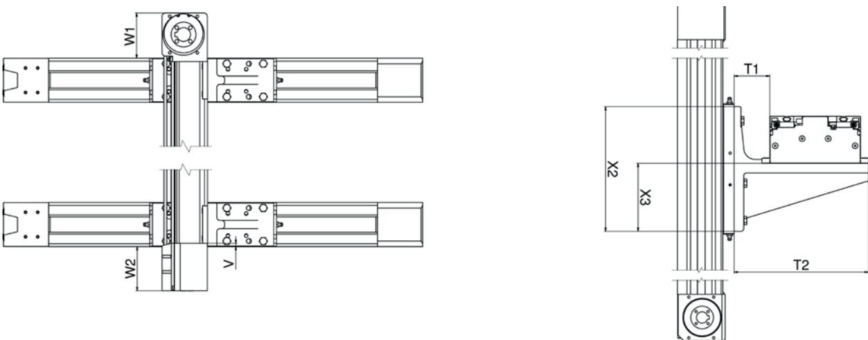
Bild 6.9 ____ Portalverbindung AXE
