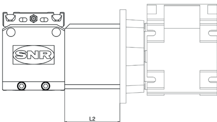
Bild 6.31 ____ Abmessungen Kupplungsglocke
