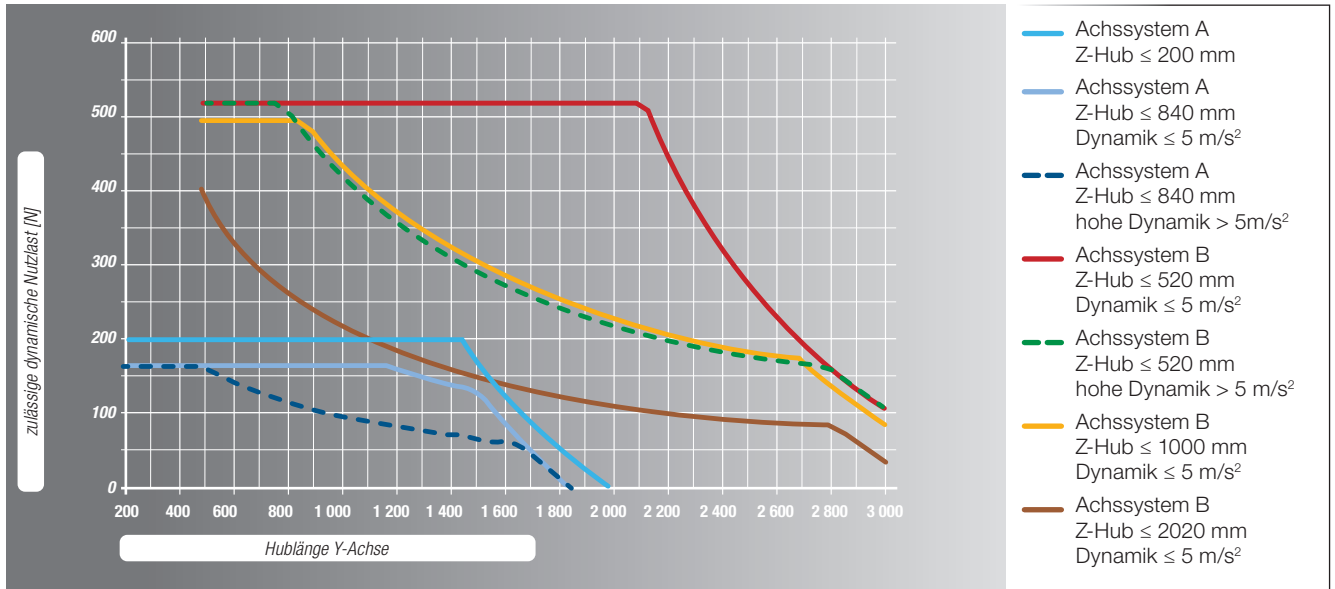
Bild 7.2 _____ dynamische Nutzlast von Standard – Achssystemen
