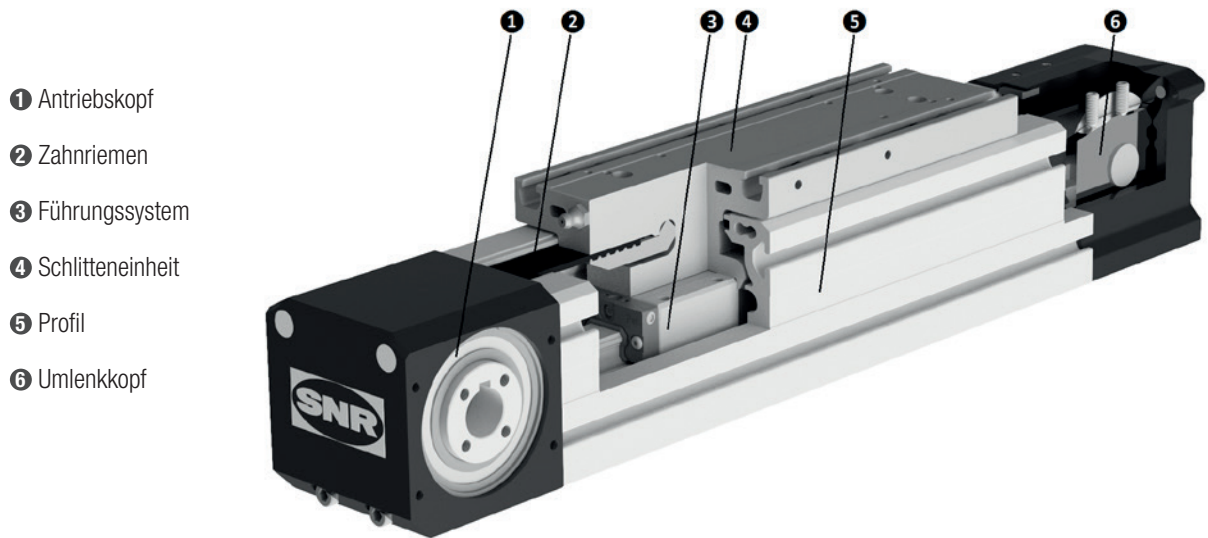
Bild 5.3 ____ Aufbau AXE60Z, AXE80Z, AXE100Z
