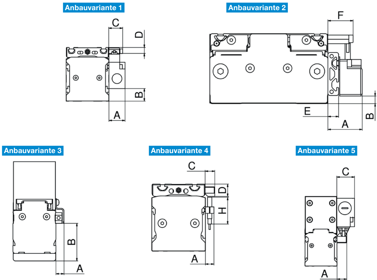
Bild 6.35 ____ Anbauvarianten der Endschalter
