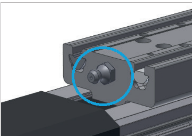
Bild 1.4 ____ Schlitteneinheit mit einer Schmierstelle stirnseitig
