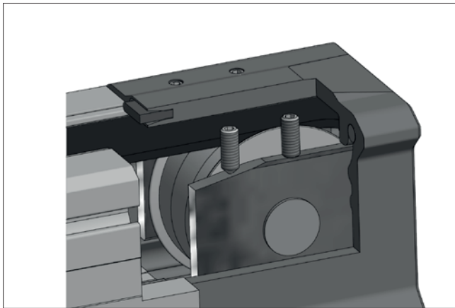
Bild 1.8 ____ Zahnriemenspannung
