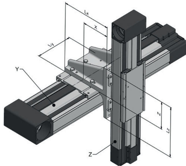
Bild 6.14 ____ Winkelverbindung Y – Z – Achs – System, Profilmontage
