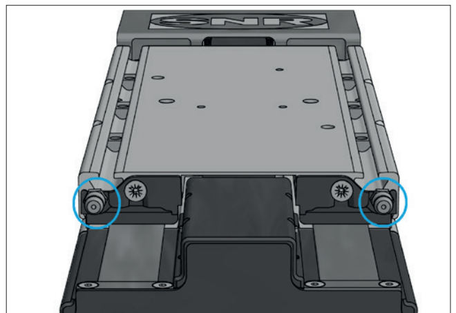
Bild 1.5 ____ Schlitteneinheit mit zwei Schmierstellen stirnseitig
