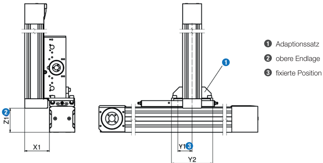
Bild 6.11 ____ A - Standardverbindung AXE
