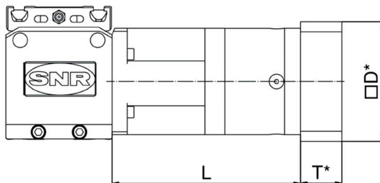
Bild 6.30 ___ Einbaumaße für kraftschlüssige Planetengetriebemontage mit Kupplung und Kupplungsglocke
