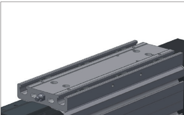
Bild 1.3 ____ Schlitteneinheit mit Profalnuten
