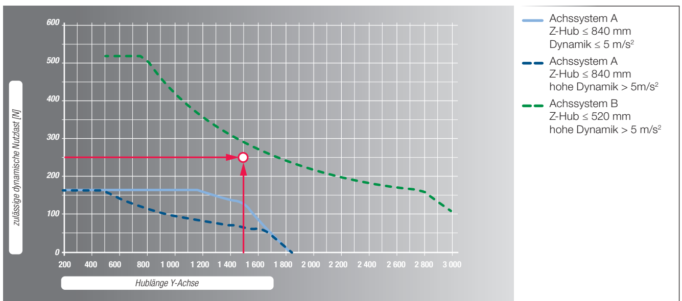
Bild 7.3 _____ dynamische Nutzlast von Standard – Achssystemen mit hoher Dynamik
