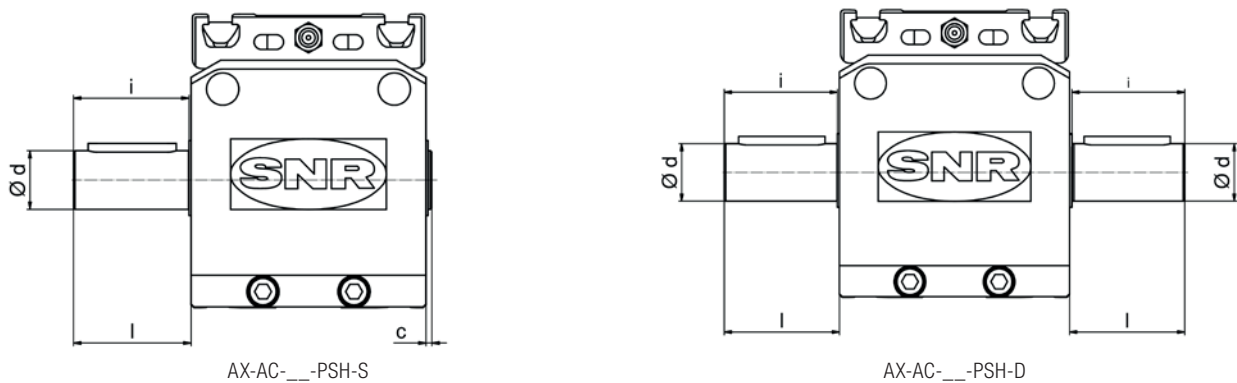
Bild 6.17 ____ Abmessungen und Anbaumaße der Steckwellen
