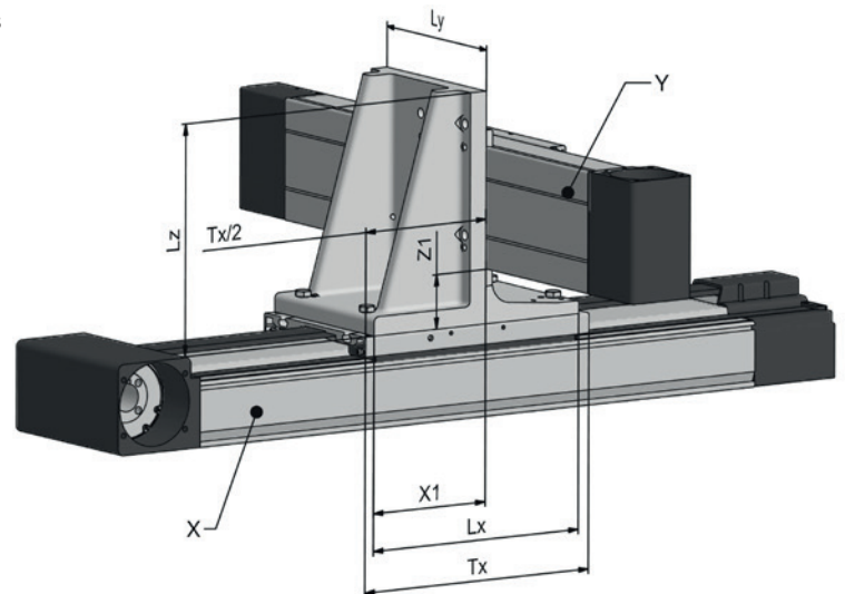
Bild 6.12 _____ Winkelverbindung X – Y – Achs – System, Profilmontage
