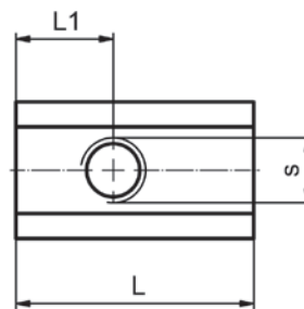
Bild 6.4 ____ Abmessungen Nutensteine
