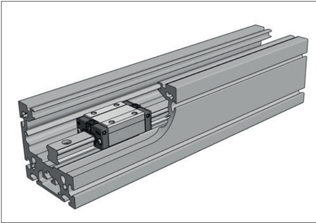
Bild 1.2 ____ Profil mit verschraubter Führungsschiene
