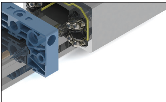
Bild 1.10 ____ SNR – Linearführung mit Kugelmutter
