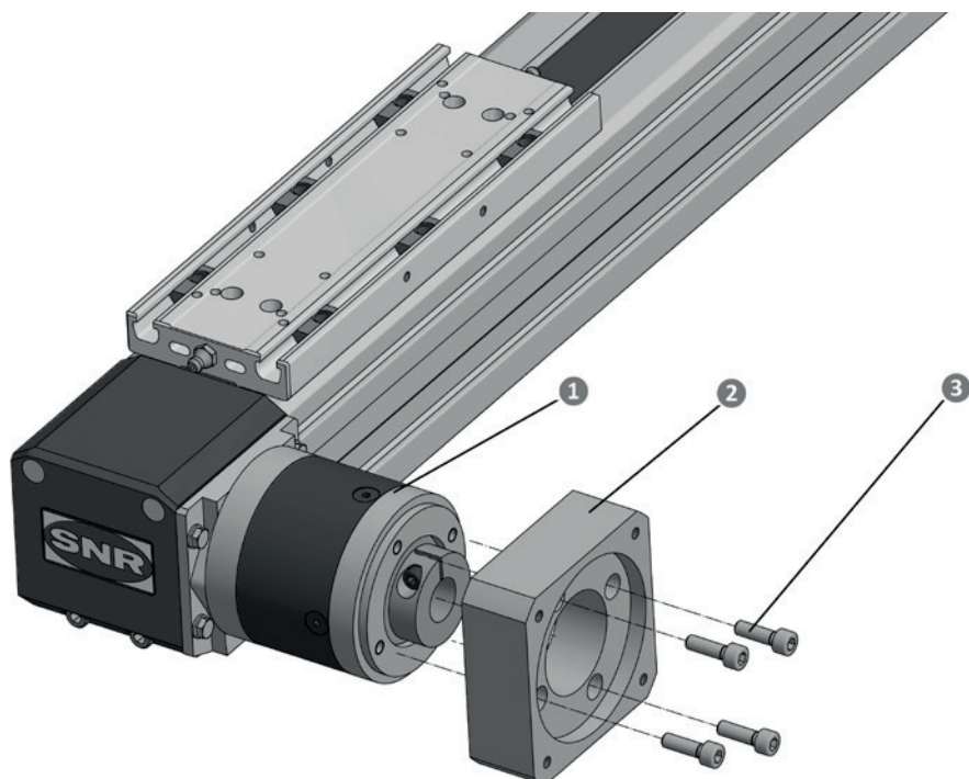
Bild 3.9 _____ Montage Getriebeflansch
