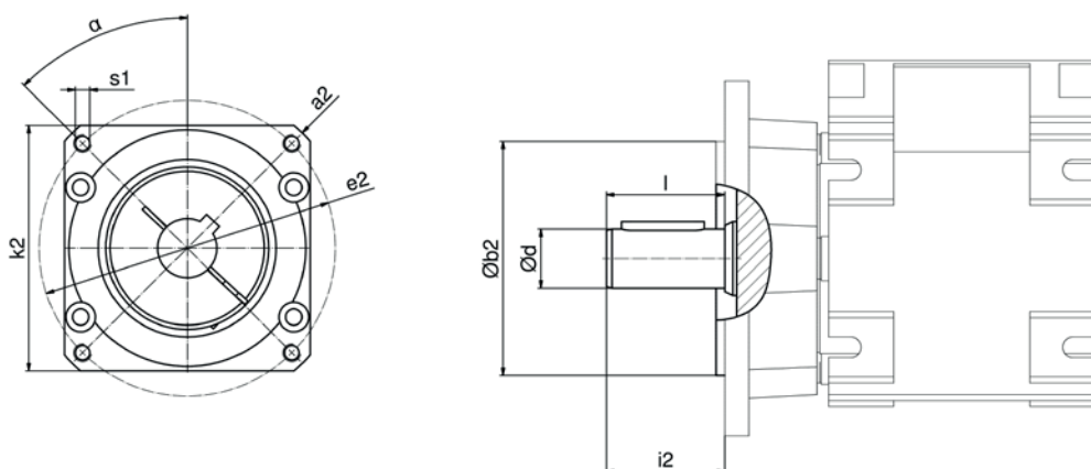
Bild 6.32 ____ Abmessungen Antriebsadaption
