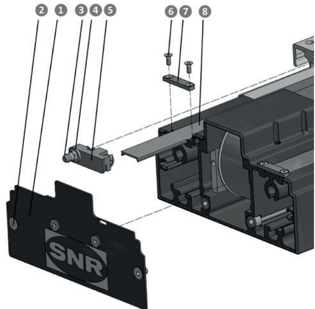
Bild 4.7 _____ Austausch Abdeckband
