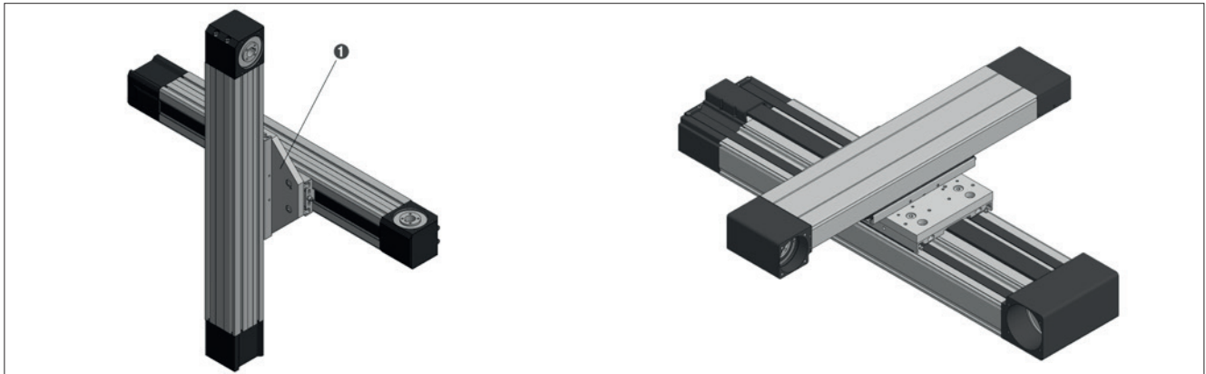
Bild 6.6 ____ Kreuzverbindung AXE
