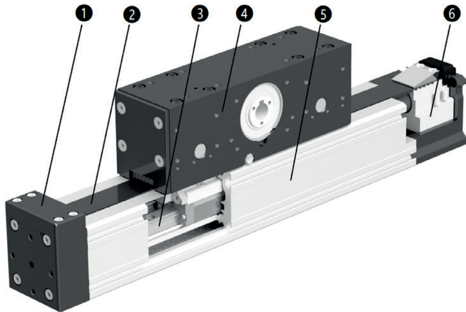
Bild 5.5 _____ Aufbau AXE_A
