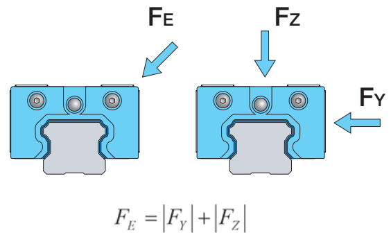
Bild 2.2 ____ Äquivalente Belastung
