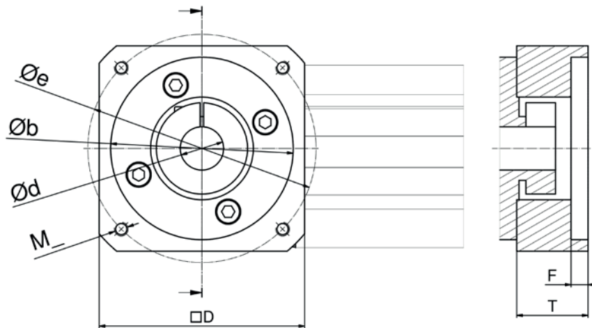
Bild 6.28 ____ Abmessungen Motoradapter
