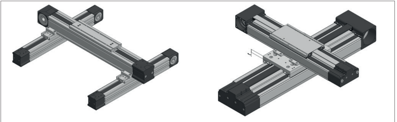
Bild 6.5 _____ Direktverbindung AXE
