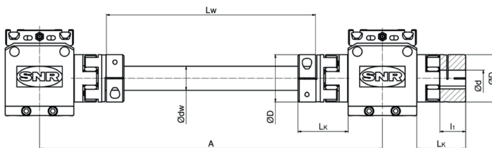
Bild 6.19 ____ Abmessungen Kupplungen und Verbindungswelle
