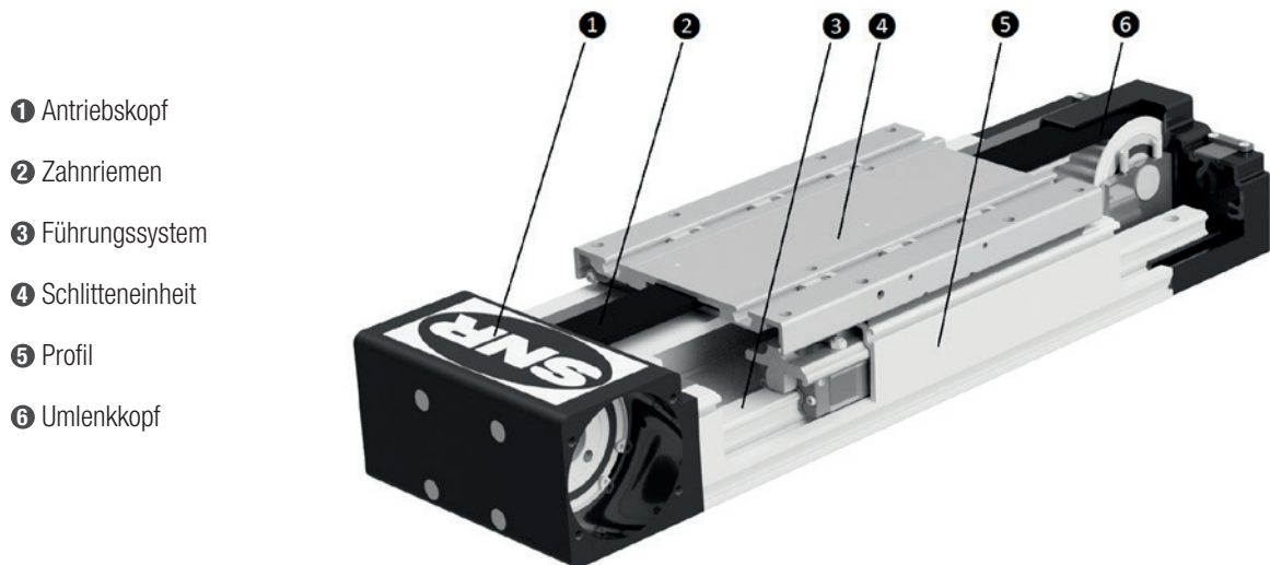
Bild 5.4 ____ Aufbau AXE110Z, AXE160Z
