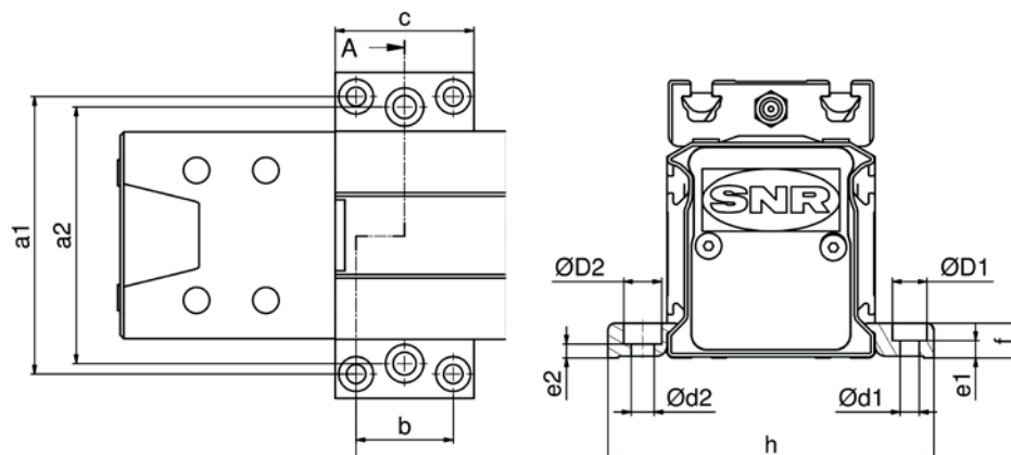
Bild 6.2 _____ Abmessungen Befestigungsleisten AXE
