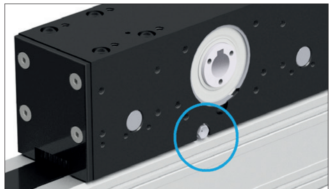
Bild 4.5 ____ Schmierstellen bei AXE40A, AXE60A
