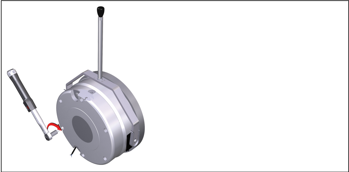
Abb. 13 Montage Magnetteil an das Lagerschild bei Doppelrotorausführung
